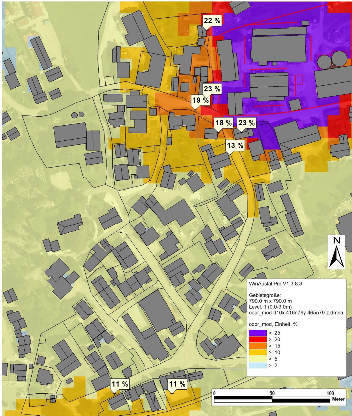
Abb. 7.1: Berechnete Gesamtbelastung für Geruch als Geruchsstundenhäufigkeit in Prozent der Jahresstunden
