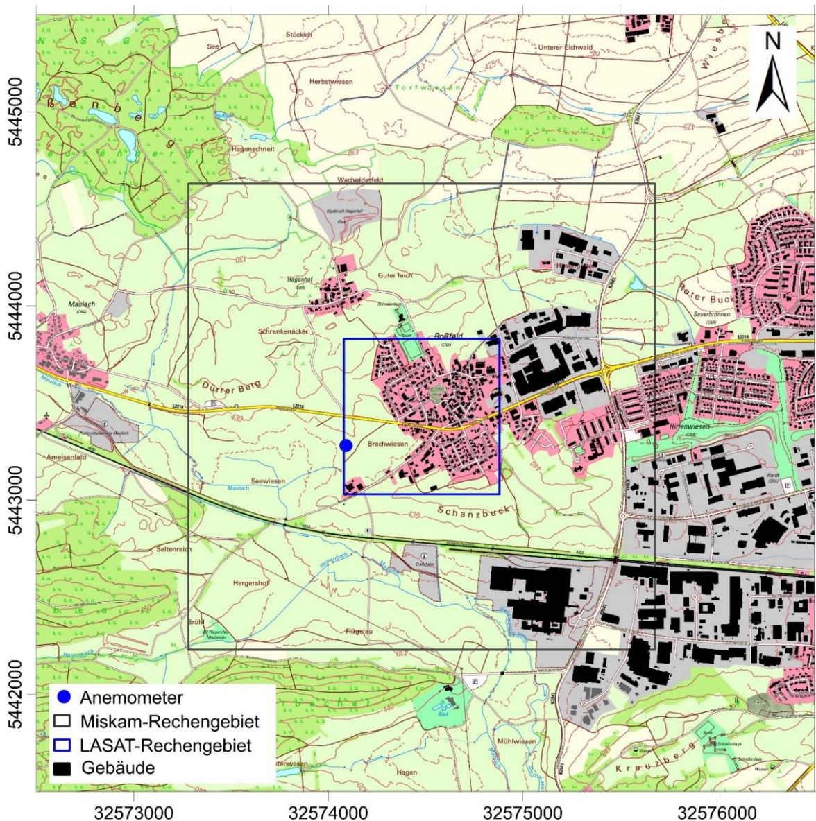
Abb. 6.1: Bei der Windfeldmodellierung mit MISKAM berücksichtigte Bebauungsstruktur (schwarz). Anemometerposition: blauer Punkt, MISKAM-Rechengebiet: äußerer grauer Rahmen, LASAT-Rechengebiet für die Ausbreitungsrechnung: blauer innerer Rahmen.
