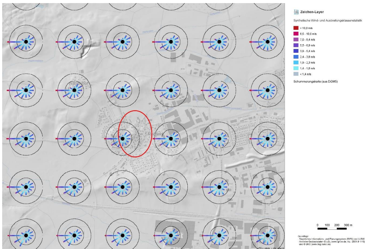
Abb. 4.6: Synthetische Windrosen in der Umgebung des Plangebiets, ergänzt um den Anlagenstandort (roter Umriss), Datenquellen: Daten aus dem UIS der LUBW
